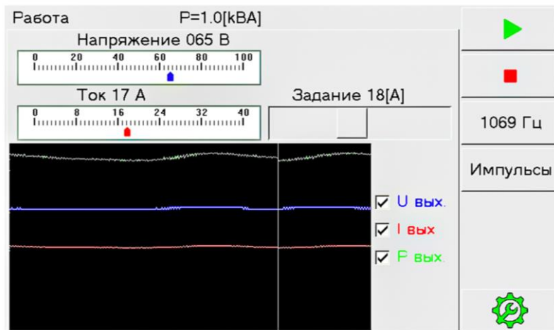
Рис.7 Показания генератора в соответствии с установленным заданием
