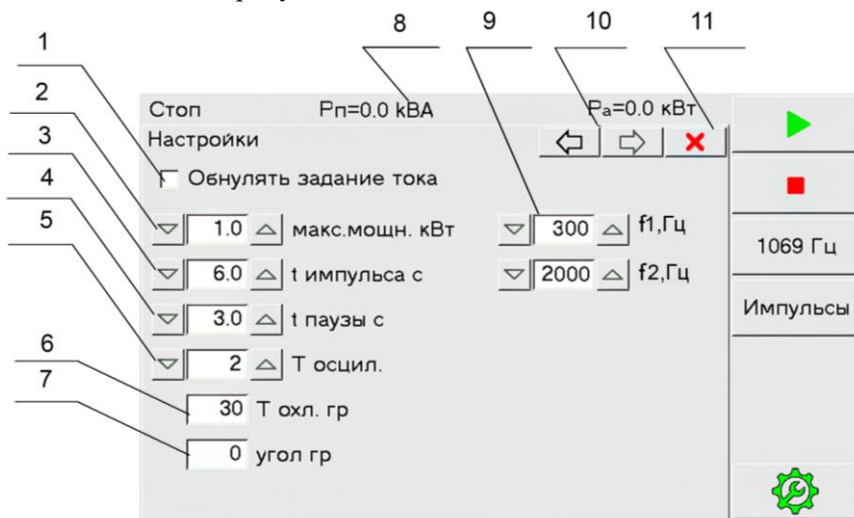
Рис.6 Меню установки и контроля параметров работы генератора
